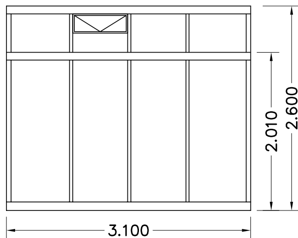
AANZICHT D
