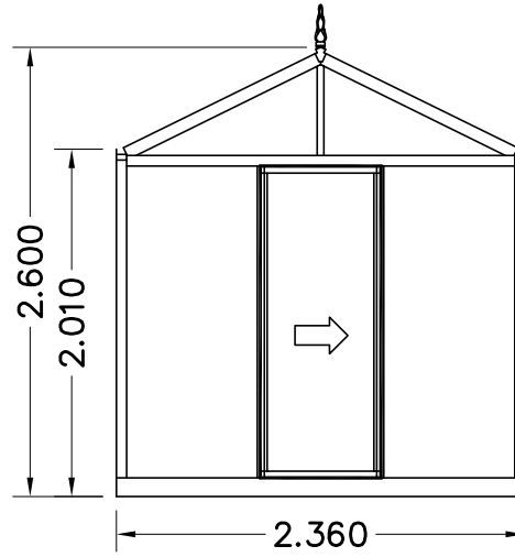
AANZICHT A
