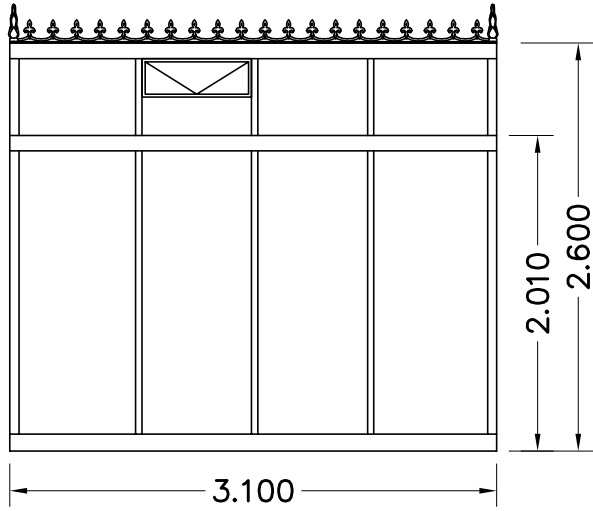
AANZICHT D
