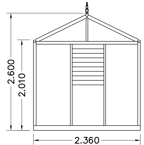
AANZICHT C
