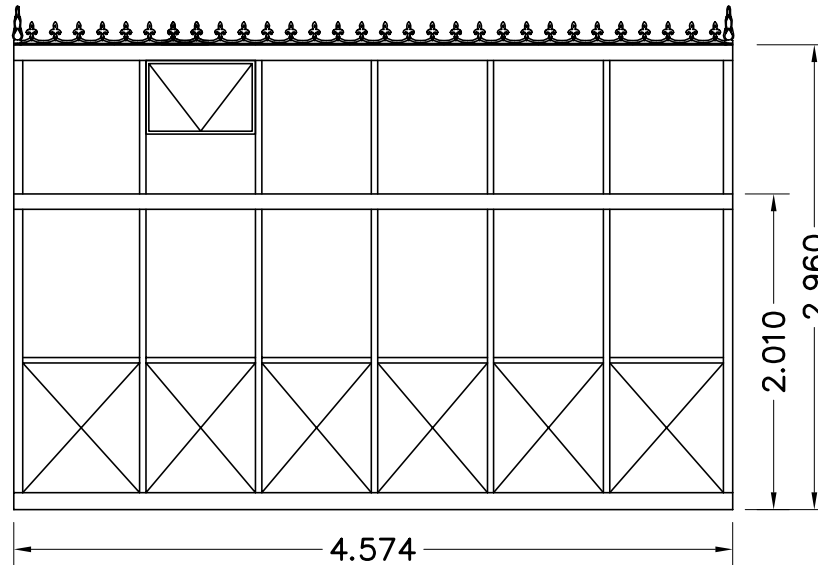
AANZICHT D
