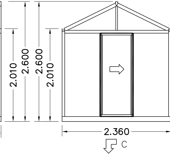
AANZICHT A
