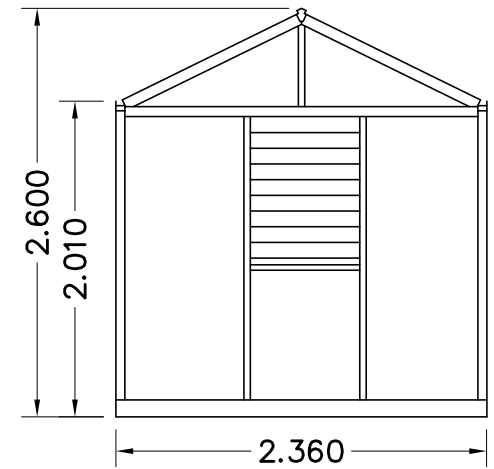
AANZICHT C
