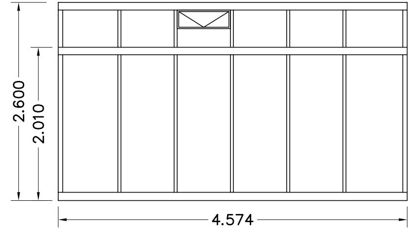
AANZICHT B
