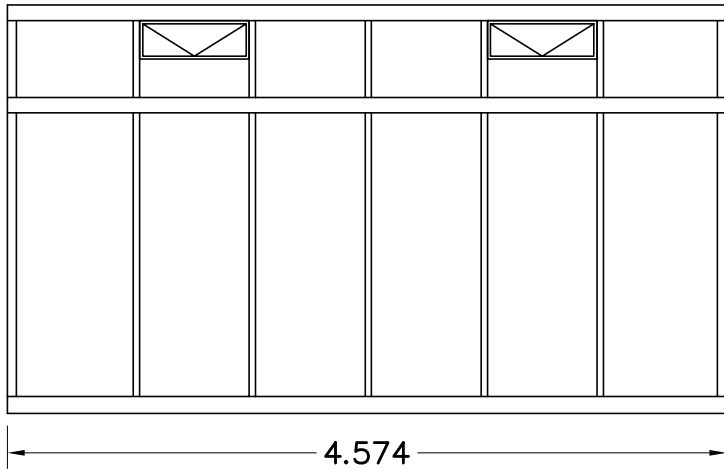
AANZICHT D
