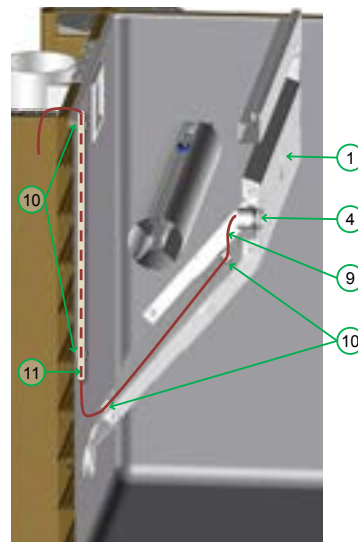
Installation des Projektorkabels
