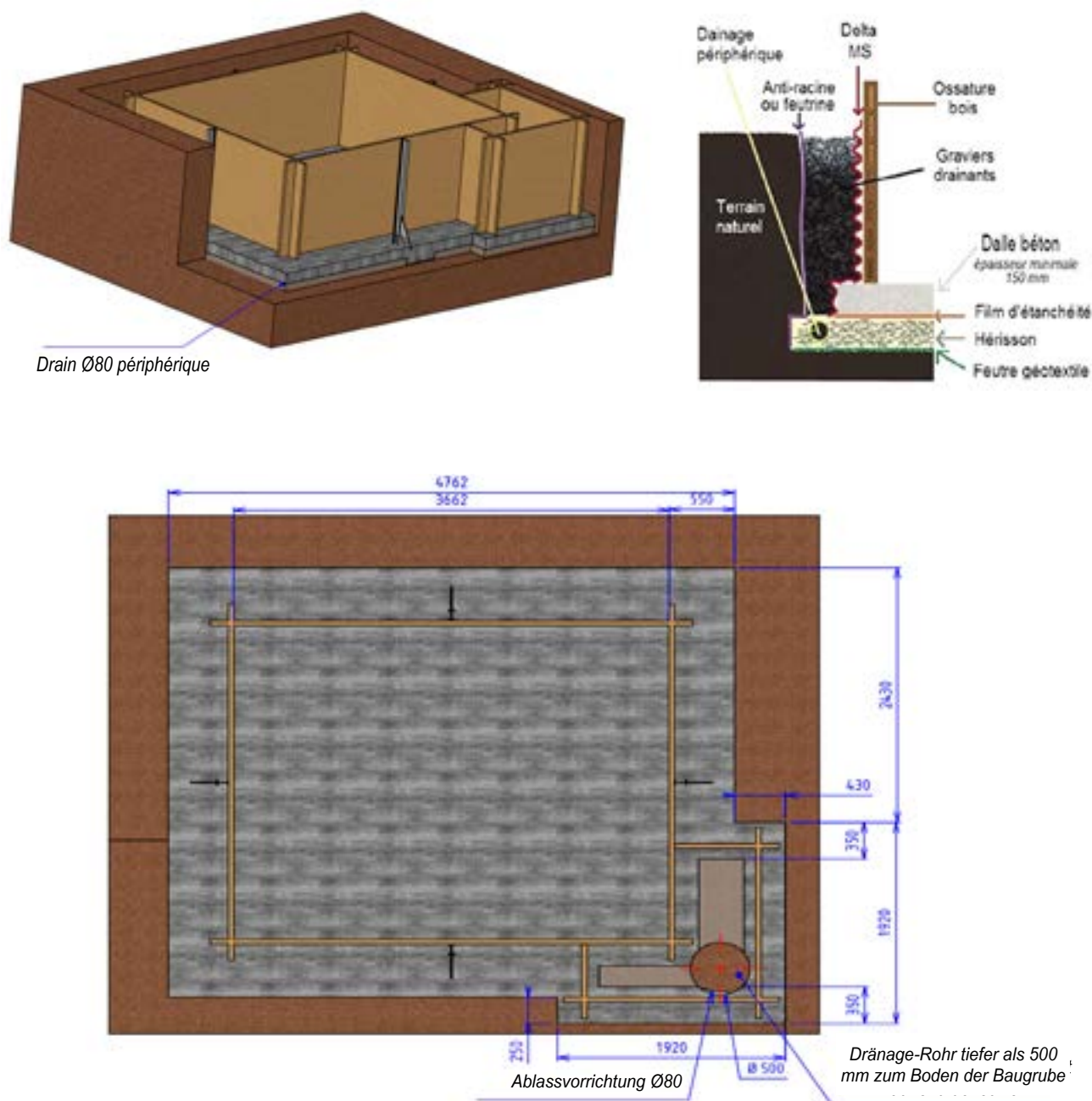
Abbildung 1 – Verlegeplan des Dränagesystems
