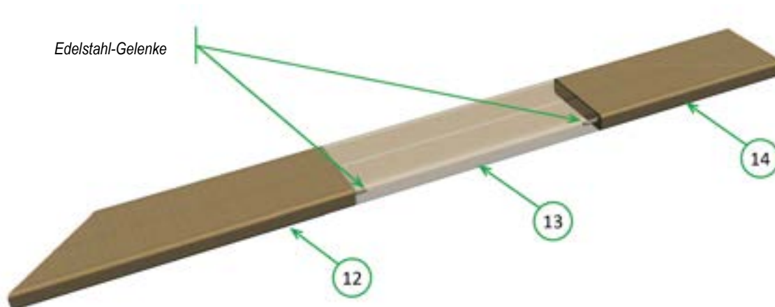
Abbildung 49 – Montage der Gelenke
