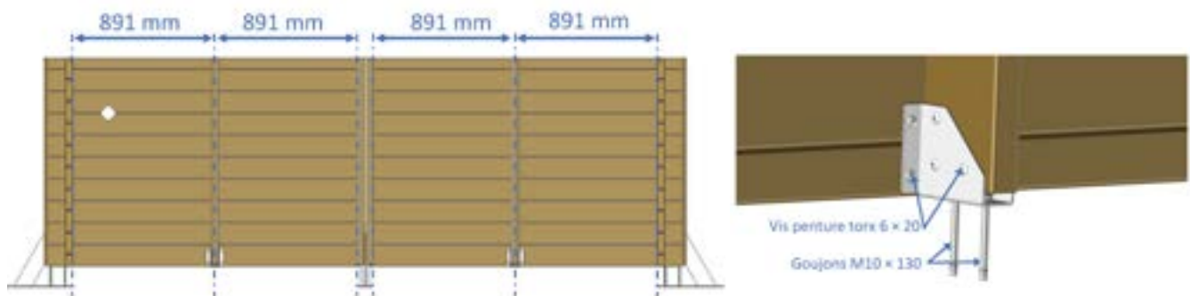
Abbildung 13 – a und b - Montage der Holzstreben
